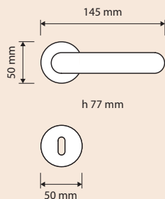
Maniglia con rosetta art.011 / Door handle on rose art.011
