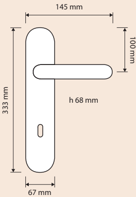
Maniglia con placca art.1770 / Door handle on plate art.1770
