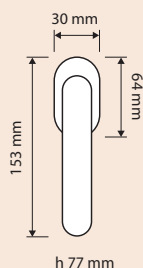
Maniglia per finestra con movimento DK 4 posizioni / Window handle with DK movement 4 clicks
