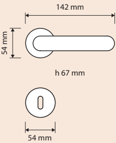
Maniglia con rosetta art.112 / Door handle on rose art.112
