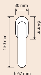
Maniglia per finestra con movimento DK 4 posizioni / Window handle with DK movement 4 clicks
