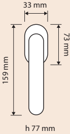
Maniglia per finestra con movimento DK SmartBlock / Window handle with DK SmartBlock movement
