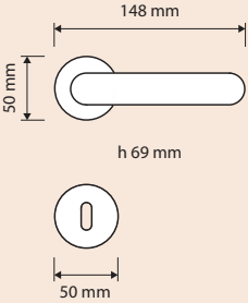
Maniglia con rosetta art.027 / Door handle on rose art.027
