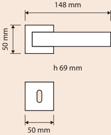
Maniglia con rosetta art.088 / Door handle on rose art.088
