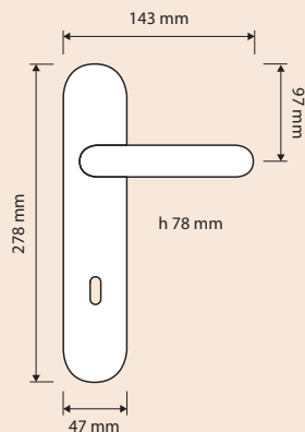
Maniglia con placca art.950 / Door handle on plate art.950
