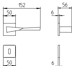
1691 maniglia per porta con rosetta door handle on rose
