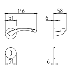
351 maniglia per porta con rosetta door handle on rose
