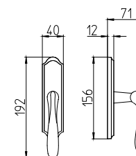
692/M cremonese window lever handle
