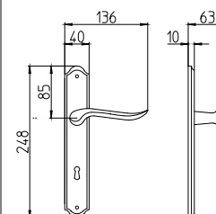
690 con piastra on backplate
