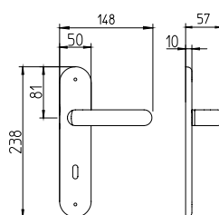
1800 con piastra on backplate
