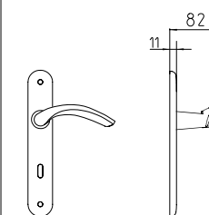
2000 con piastra on backplate
