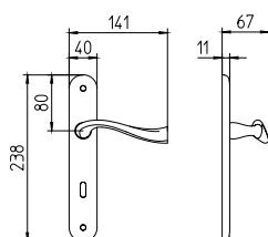
990 con piastra on backplate
