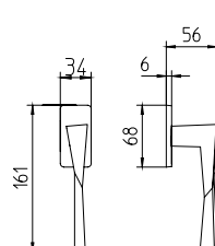
1692/DK martellina dk drehkipp system
