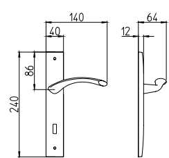
350 con piastra on backplate
