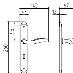
980 con piastra on backplate
