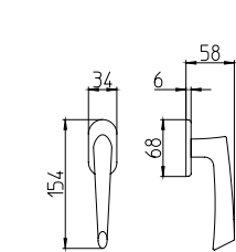
352/DK martellina dk drehkipp system
