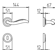
981 maniglia per porta con rosetta door handle on rose
