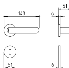
1801 maniglia per porta con rosetta door handle on rose
